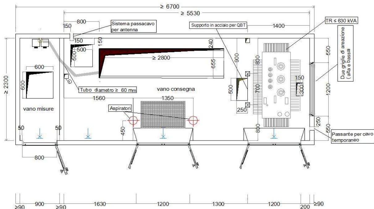
Fig. 1 – Pianta cabina consegna Utente
